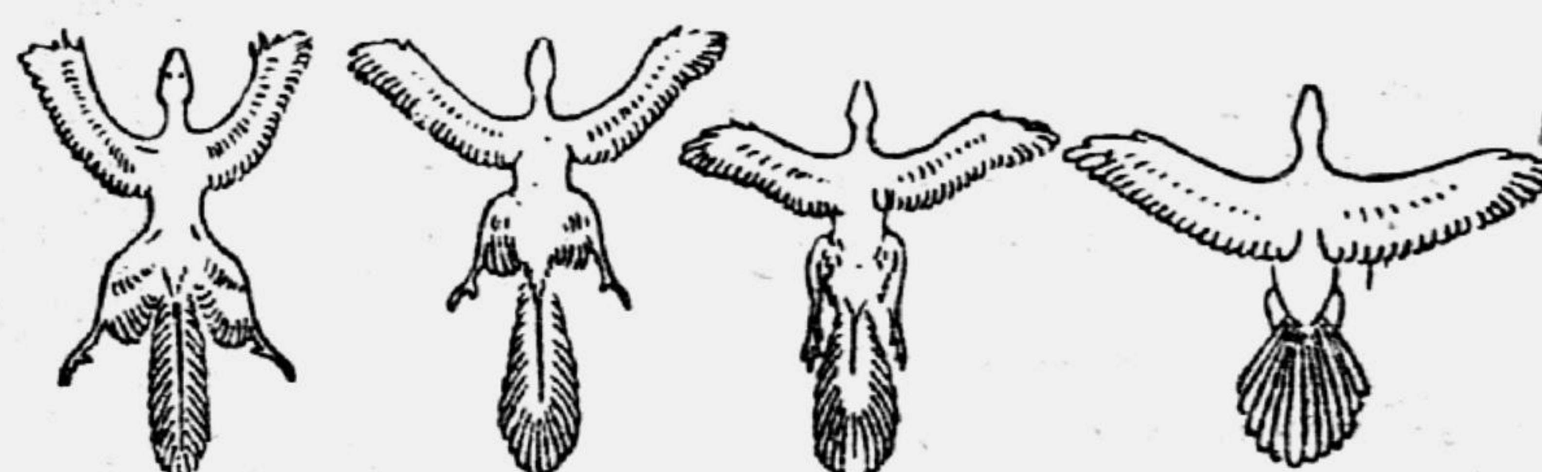
5. Предполагаемые четыре ступени в развитии полёта у птиц.
